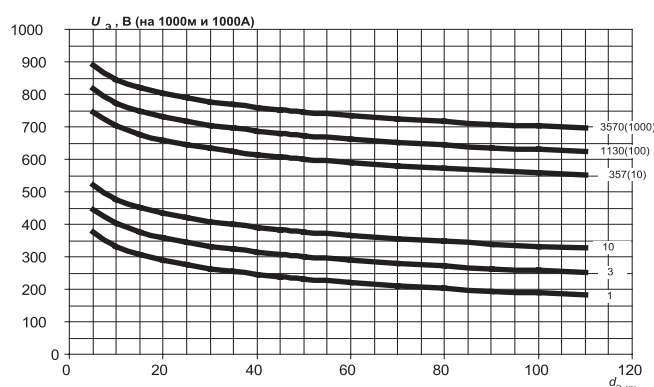
Рис. 5. Несимметричный режим. Напряжение относительно земли на экране кабеля 6–500 кВ длиной 1000 м при токе жилы 1000 А в зависимости от диаметра экрана d_\Omega и глубины D_\Omega
