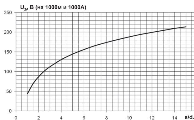
Рис. 4. Симметричный режим. Напряжение относительно земли на экране кабеля 6–500 кВ длиной 1000 м при токе жилы 1000 А в зависимости от соотношения s/d_\Omega
